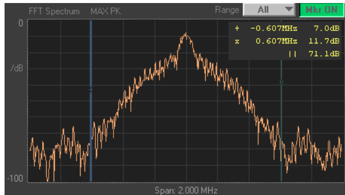
Fig. 45: FFT spectrum display
