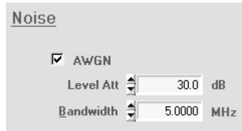
Fig. 10: AWGN settings
